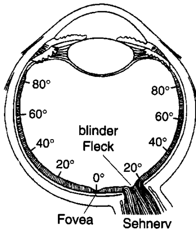
4.6 Die Verteilung von Stäbchen und Zapfenrezeptoren in der Netzhaut Dargestellt ist die Dichte der Stäbchen und Zapfen für einen horizontalen Schnitt durch das linke Auge in Höhe der Fovea und des blinden Flecks als Funktion des Abstandes (in Grad) vom Zentrum der Fovea.
