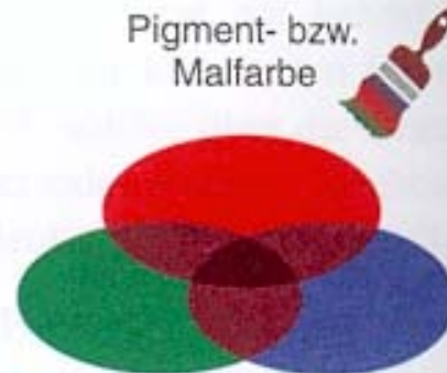
subtraktive Farbmischung
