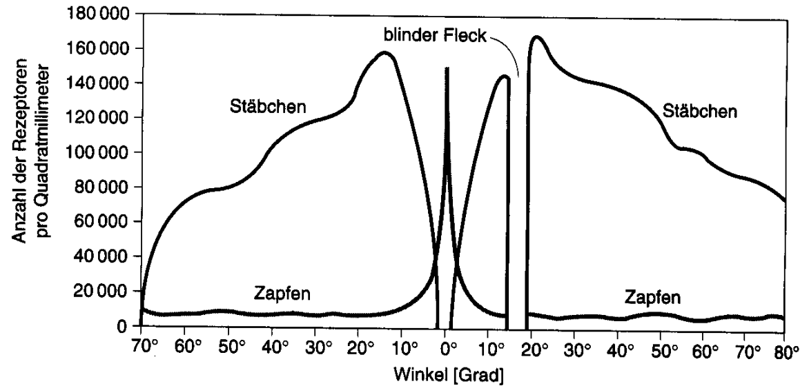
4.6 Die Verteilung von Stäbchen und Zapfenrezeptoren in der Netzhaut Dargestellt ist die Dichte der Stäbchen und Zapfen für einen horizontalen Schnitt durch das linke Auge in Höhe der Fovea und des blinden Flecks als Funktion des Abstandes (in Grad) vom Zentrum der Fovea.
